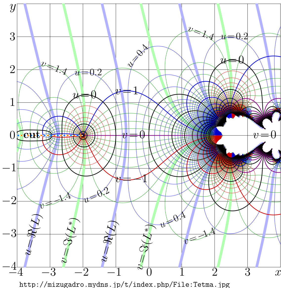
Fig. 14.12: u+iv=\text{tet}(x+iy) [tetmap]
