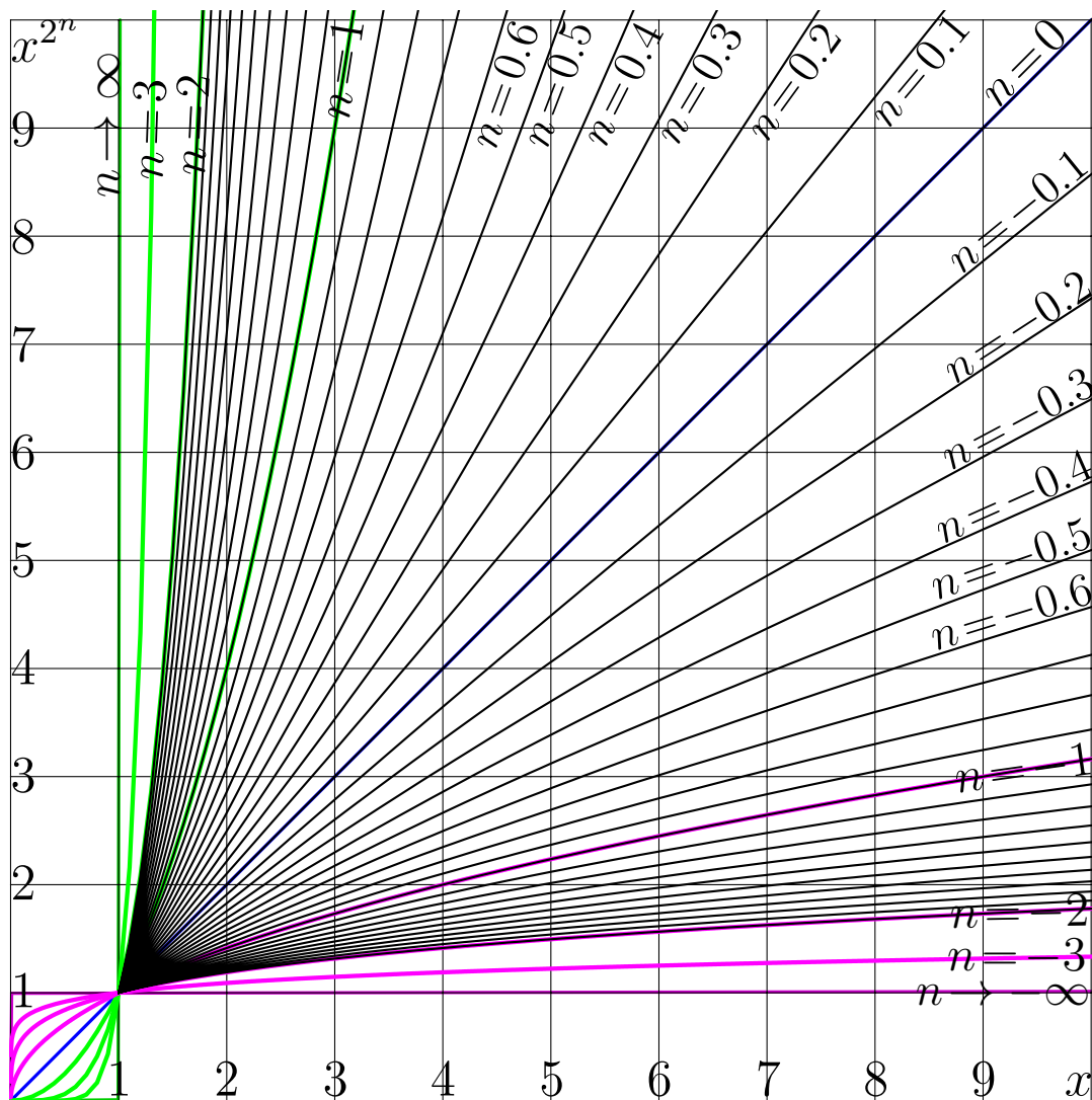
Fig. 4.13: y = T^n(x) = \text{Pow}_2^n(x) для различных n . [IterPowPlot]
