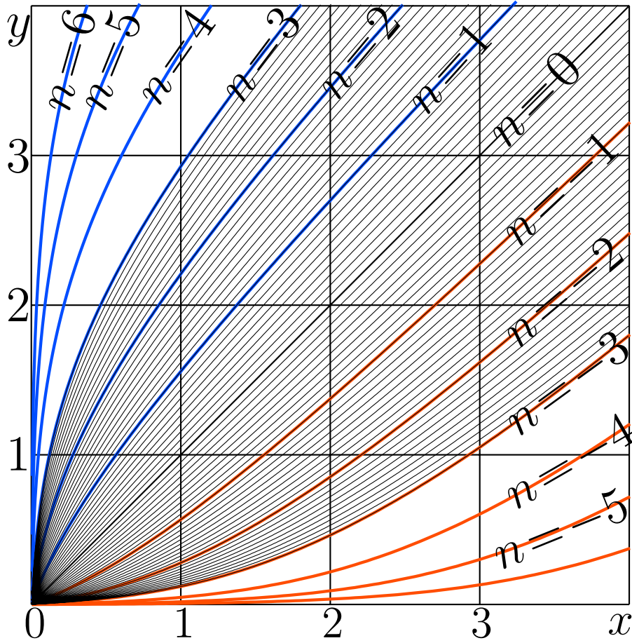
Fig. 5.6: y = \text{Doya}^n(x) по формуле (5.13) [doyaplo]
