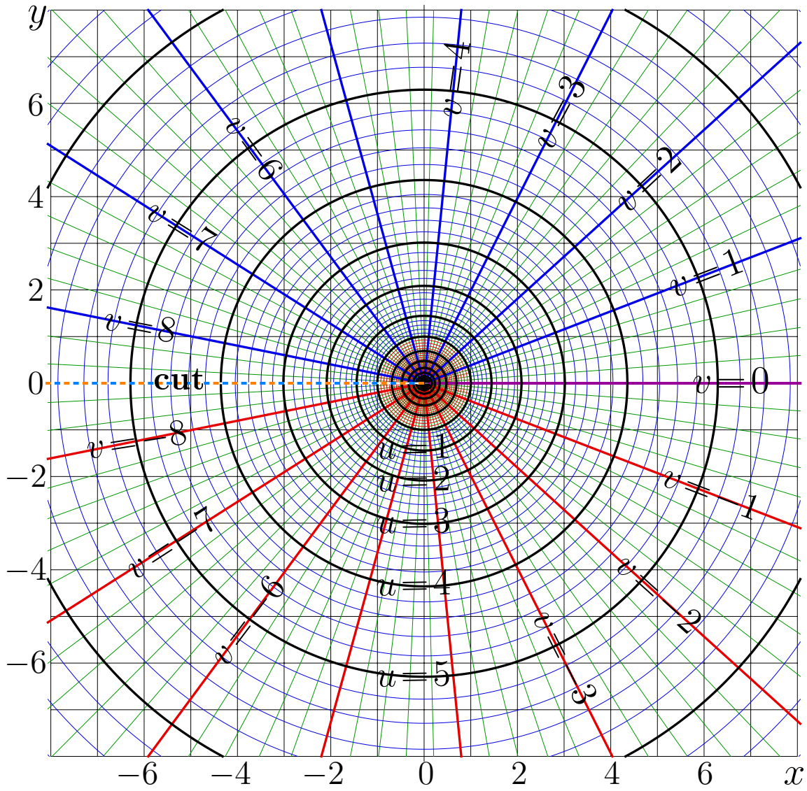
Fig. 10.4: u+iv=\log_{\eta}(x+iy)
