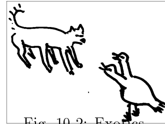
Fig. 10.2: Exotics
