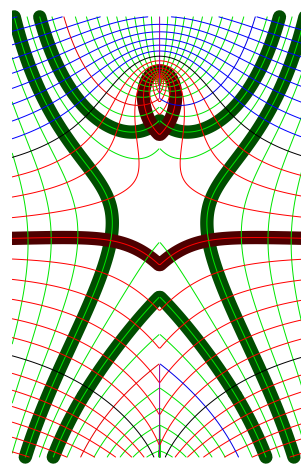
Fig. 5.14: Eureka!
